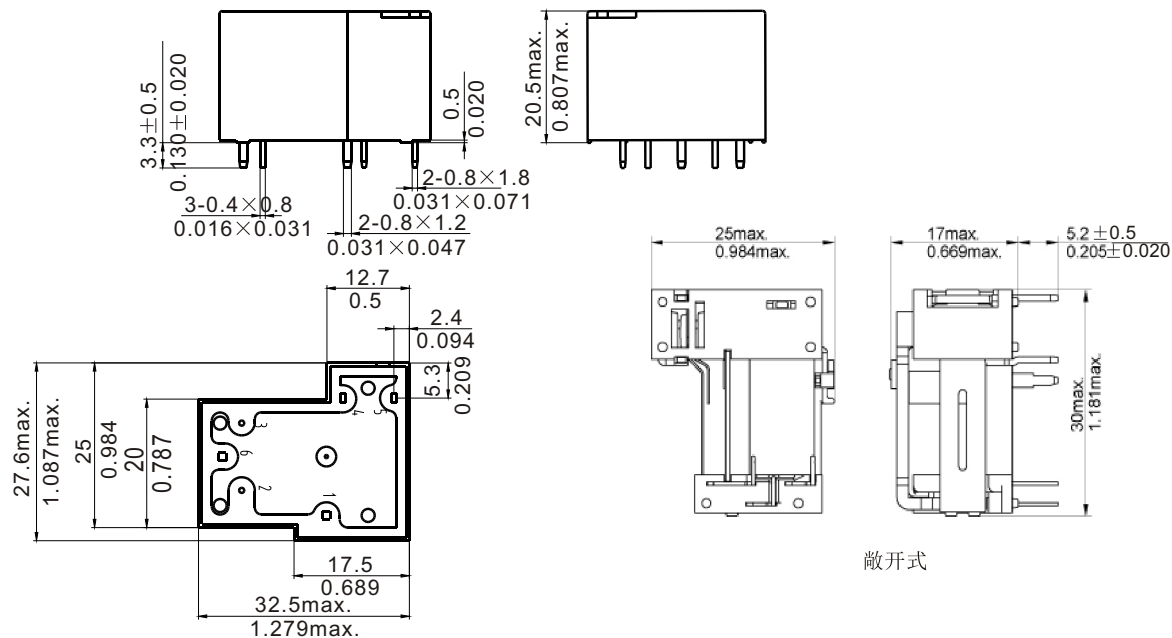
外形尺寸图
